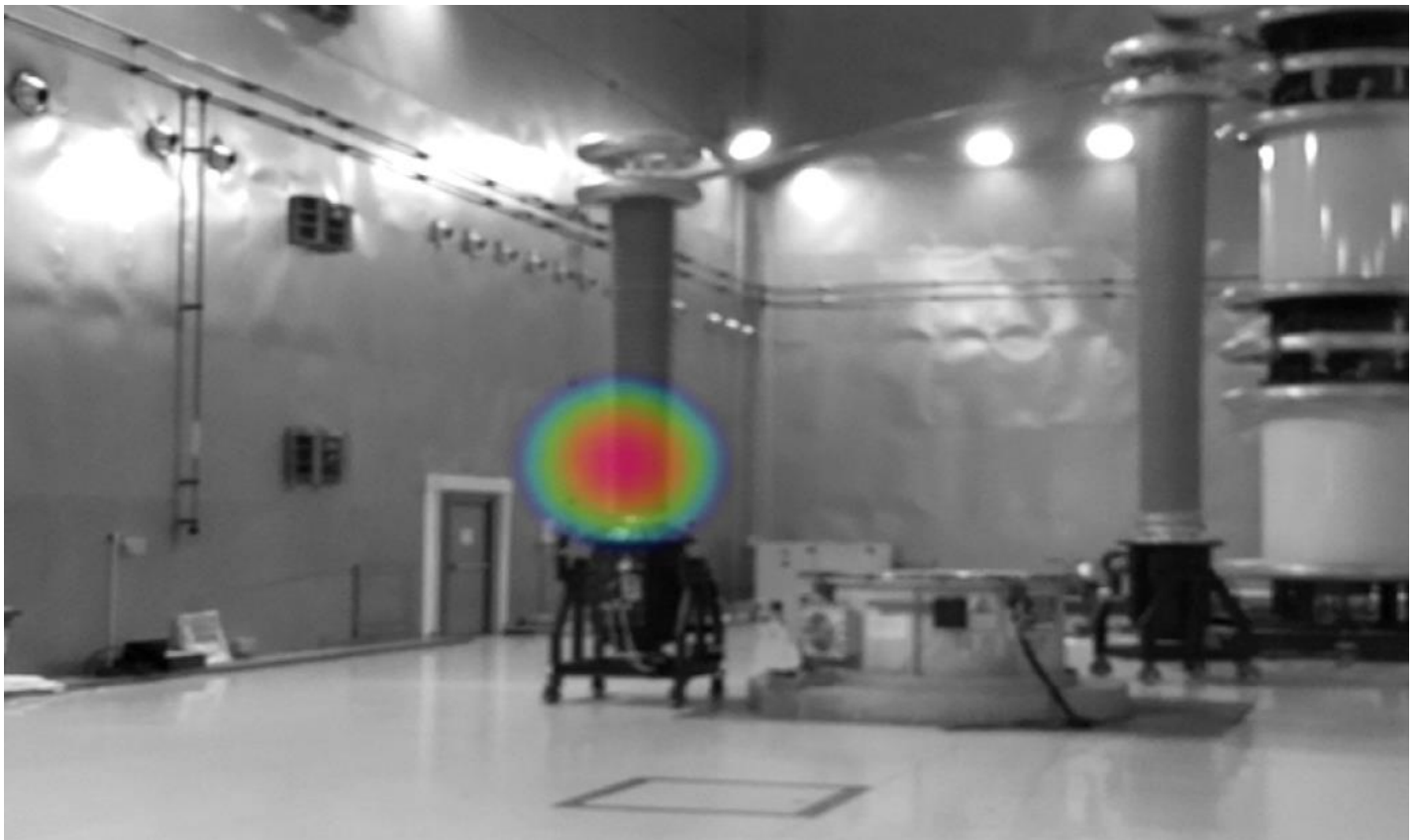
Imagem 2. Outro instantâneo do laboratório HV mostra a superfície ou descarga interna em uma bucha.
