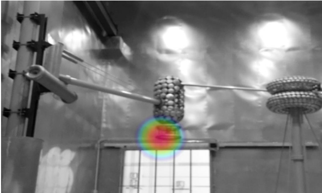
Imagem 1. A câmera NL encontrou descarga corona negativa em um eletrodo anticorona no laboratório de teste da Grid Solutions & GE Renewable Energy Italy.
