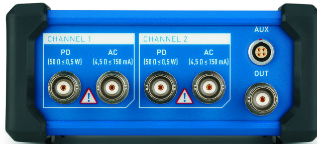
Figura 2-3: Painel traseiro do sistema de medição MPD 800
